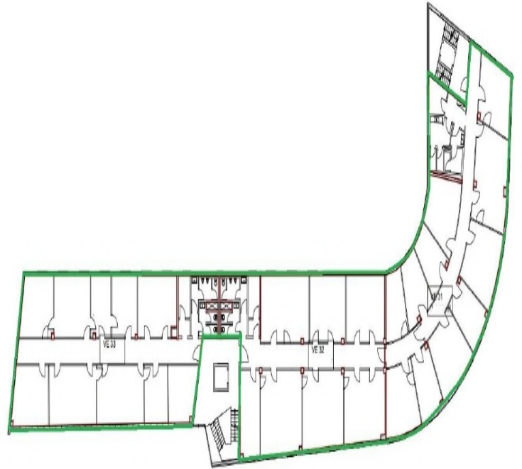
3. Obergeschoss
