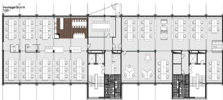
Grundriss Musterplanung Regelgeschoss
